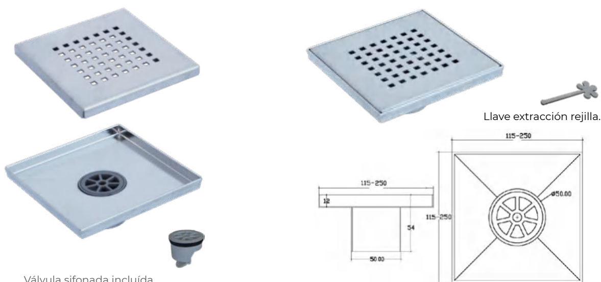
Válvula sifonada incluida.
